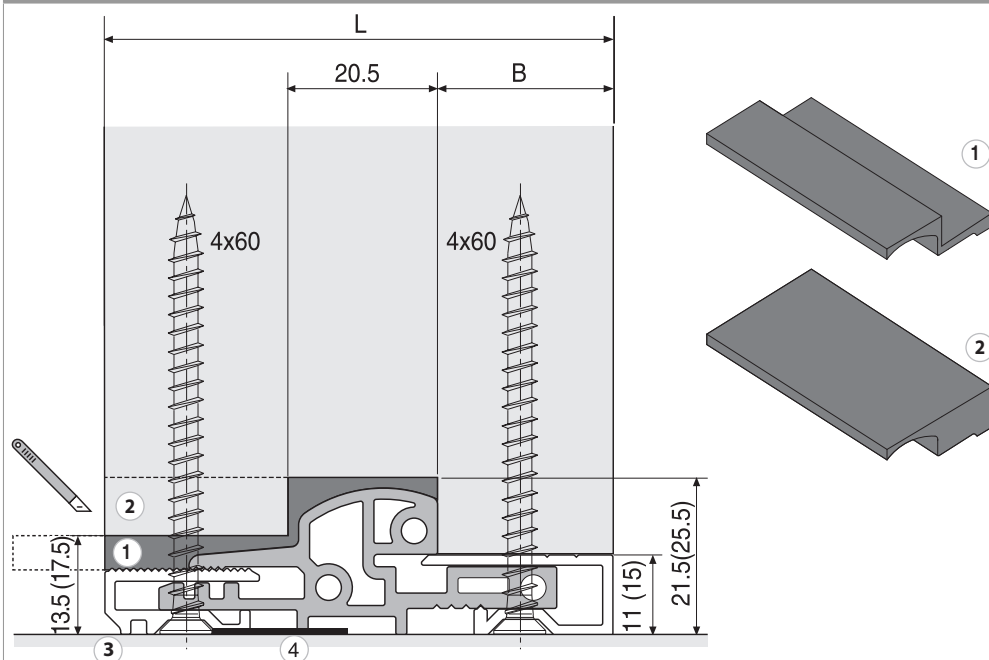
Schnitt Stock
