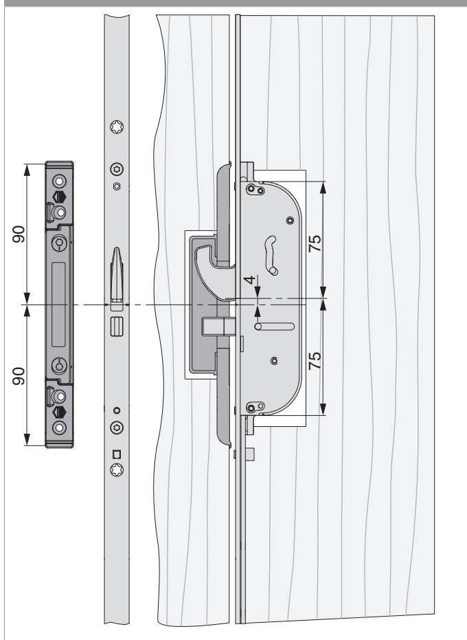
Schließteile Haken-Bolzen
