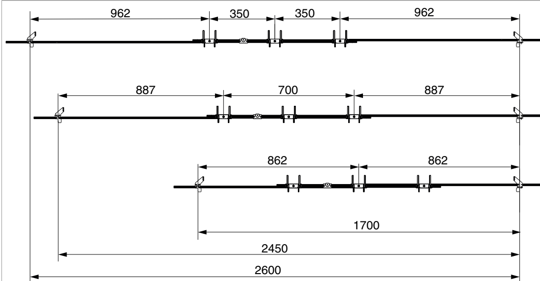
Schließteilpositionen mit Lehre 57247
