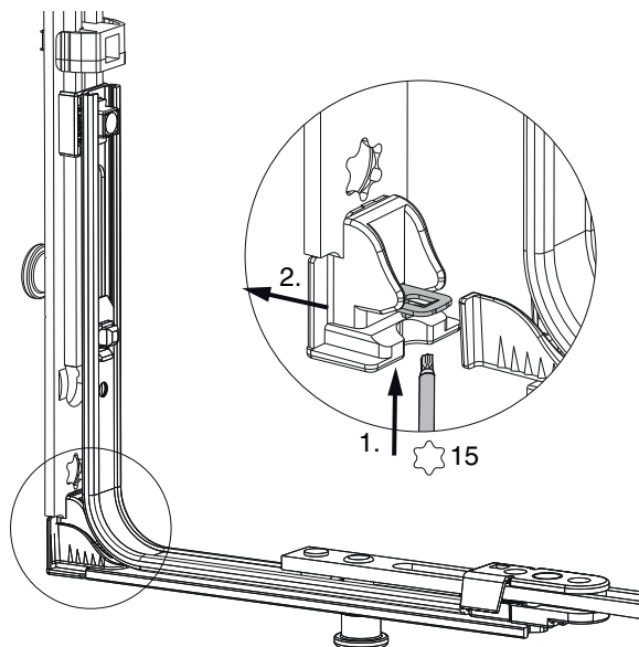
Klipsverbindung aushängen
