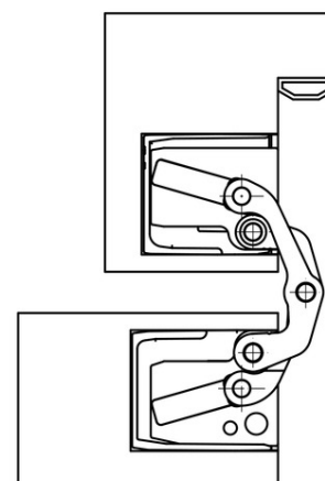
Rámová zárubeň 180°
